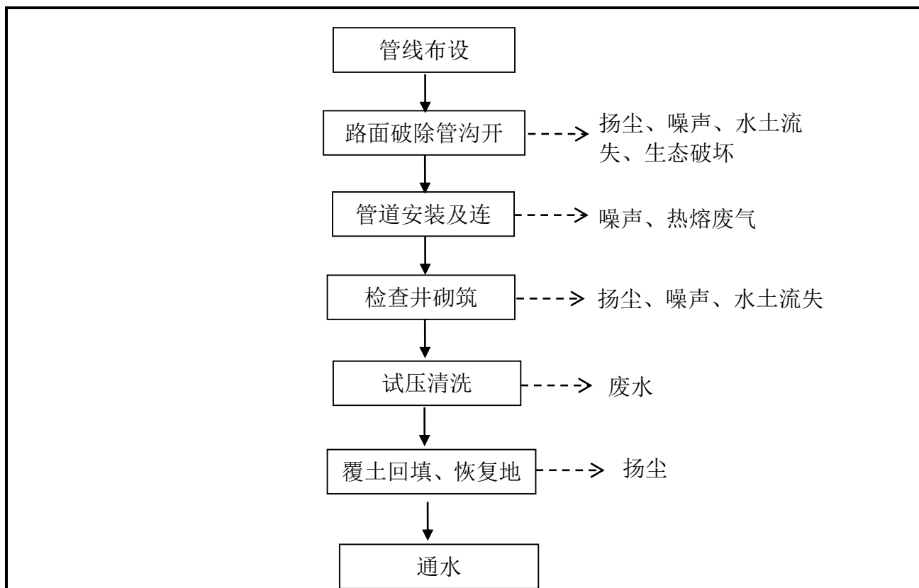
图 4-1 管网施工工艺流程及产污环节图
