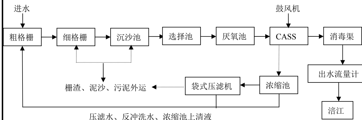
图 3-1 松垭污水处理厂工艺流程图
